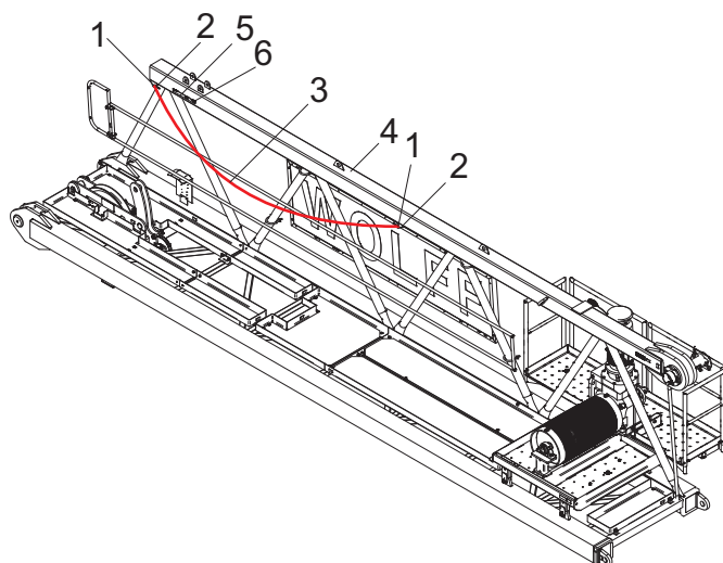
Anschlageinrichtung am Ausleger; Auslegerstück 1 innen; Teile zur besseren Ansicht ausgeblendet
