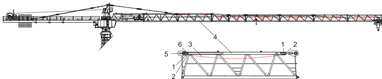
Anschlageinrichtung am Ausleger (exemplarisch)
