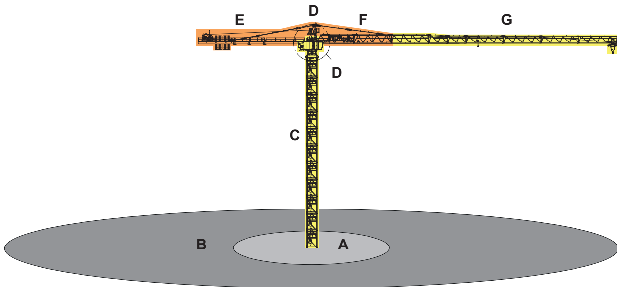
Gefahrenbereiche am Turmdrehkran
