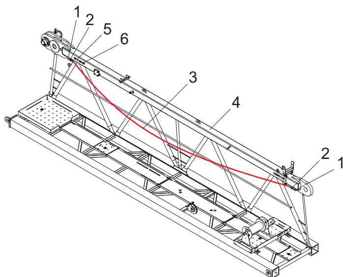
Anschlageinrichtung am Ausleger; Auslegerstück 2 innen, Teile zur besseren Ansicht ausgeblendet
