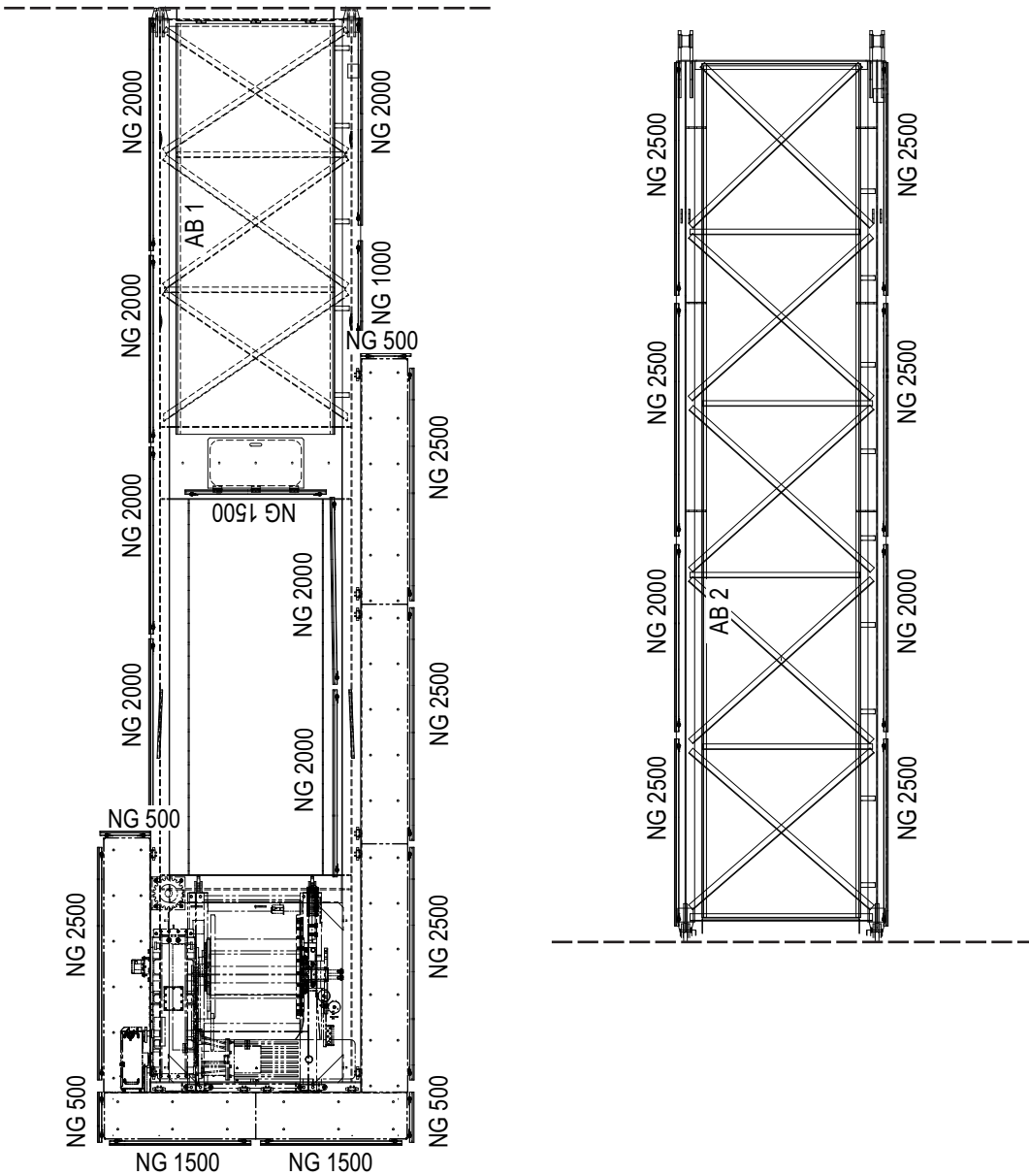
Normgeländeranordnung Gegenausleger
