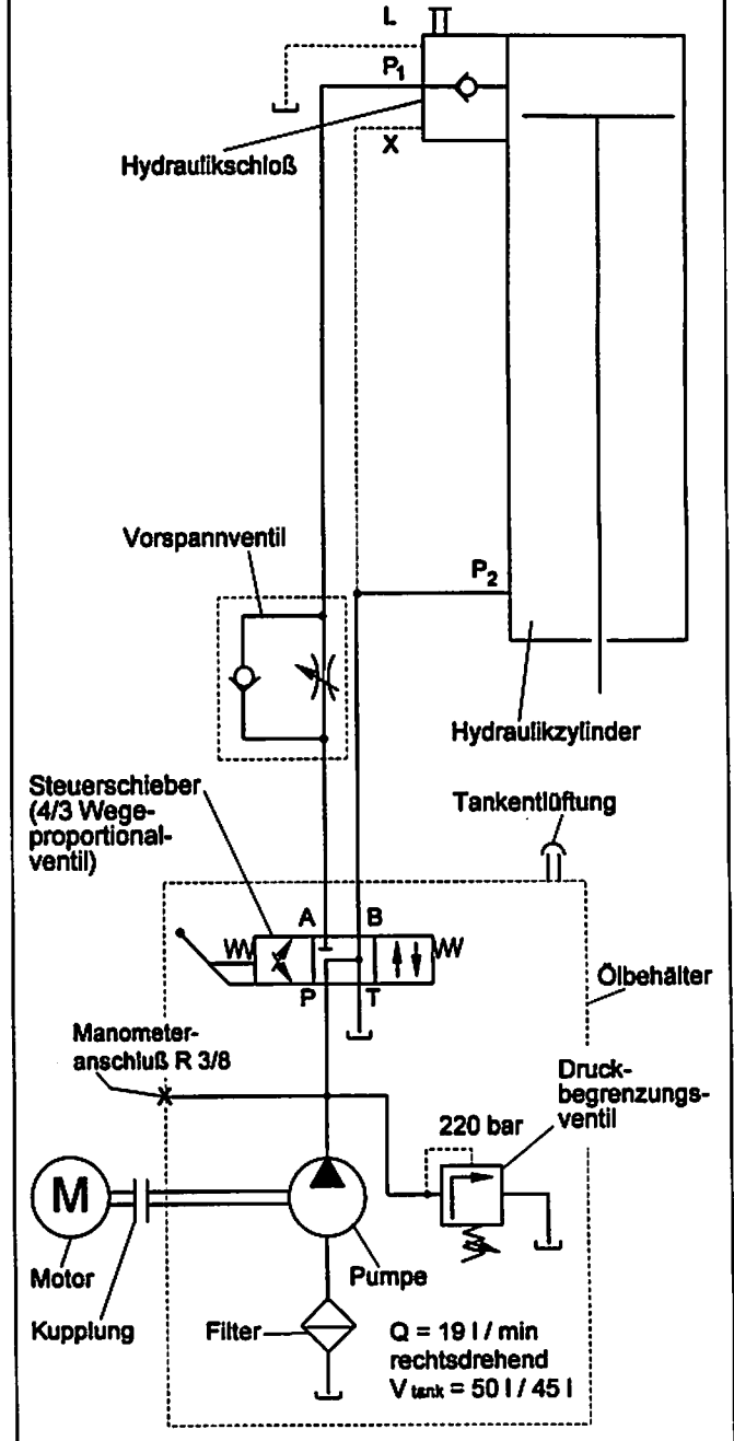
Hydraulikschema
