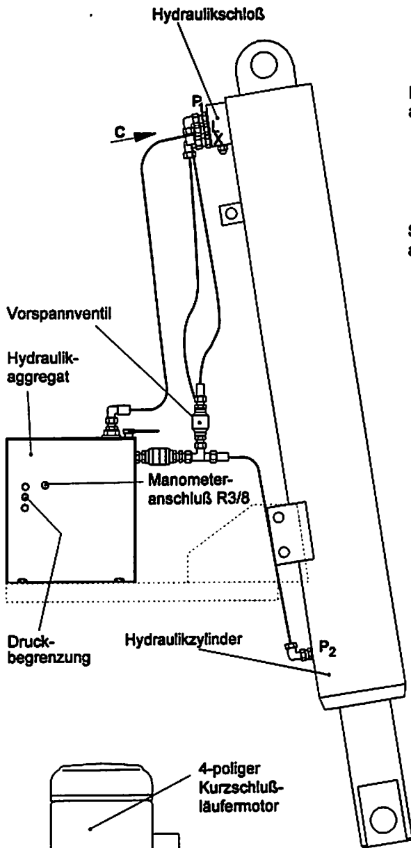
Hydraulikschema
