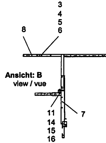
Leiterverlängerung (Pos.8) für Fundamentkreuz 91EC in Pos. ① ladder extension for cruciform base 91EC in pos. ① / échelle rallonge pour châssis en croix 91EC en pos. ①
