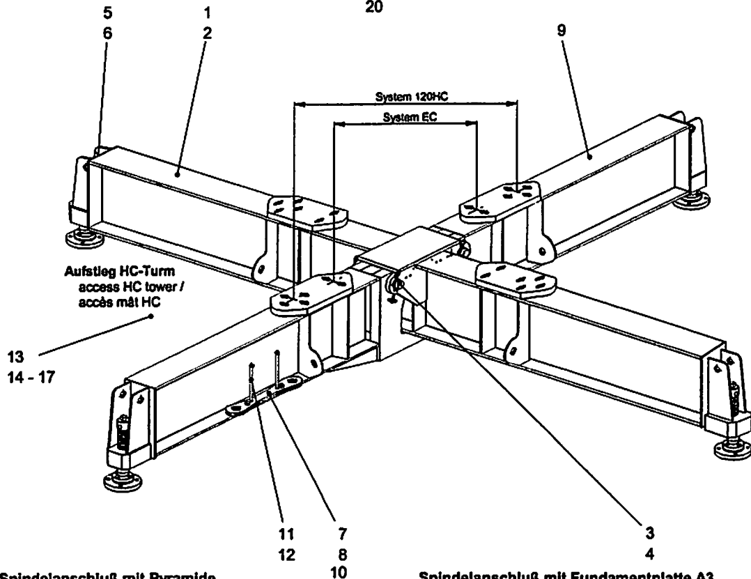
Spindelanschluß mit Pyramide outrigger jack connection with pyramidal support raccord du vérin mécanique avec support pyramidal
