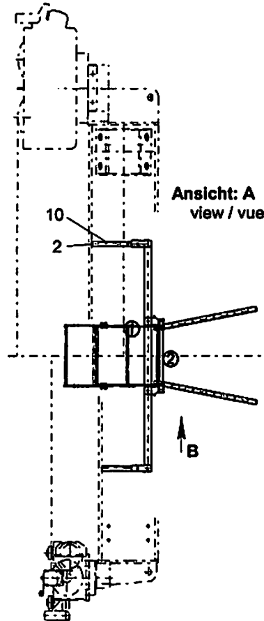
Leiterverlängerung (Pos.8) für Fundamentkreuz 71EC in Pos. ② ladder extension for cruciform base 71EC in pos. ② / échelle rallonge pour châssis en croix 71EC en pos. ②
