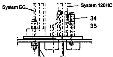
Befestigung der Turmstücke fastening of tower sections / fixation des éléments de mât
