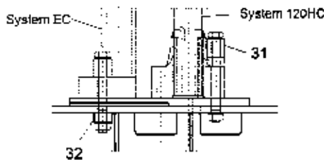
Befestigung der Turmstücke fastening of tower section / fixation des éléments de mâât
