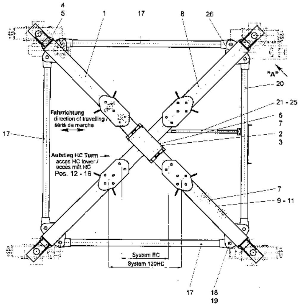
Befestigung der Turmstücke fastening of tower section / fixation des éléments de mâât
