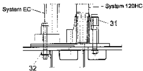
Befestigung der Turmstücke fastening of tower section / fixation des éléments de mât
