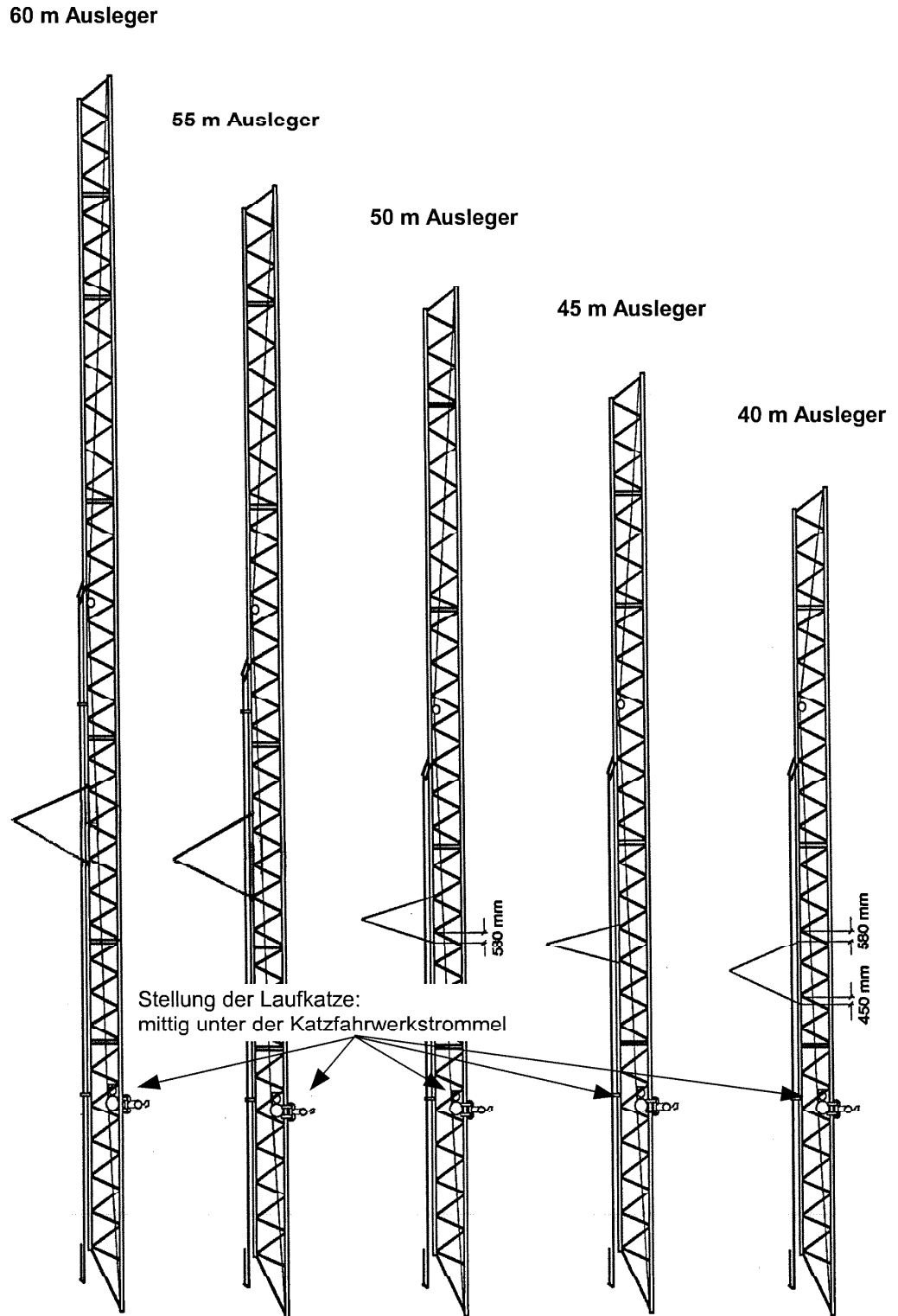
Fig. 6-22 Anschlagpunkte des Auslegers
