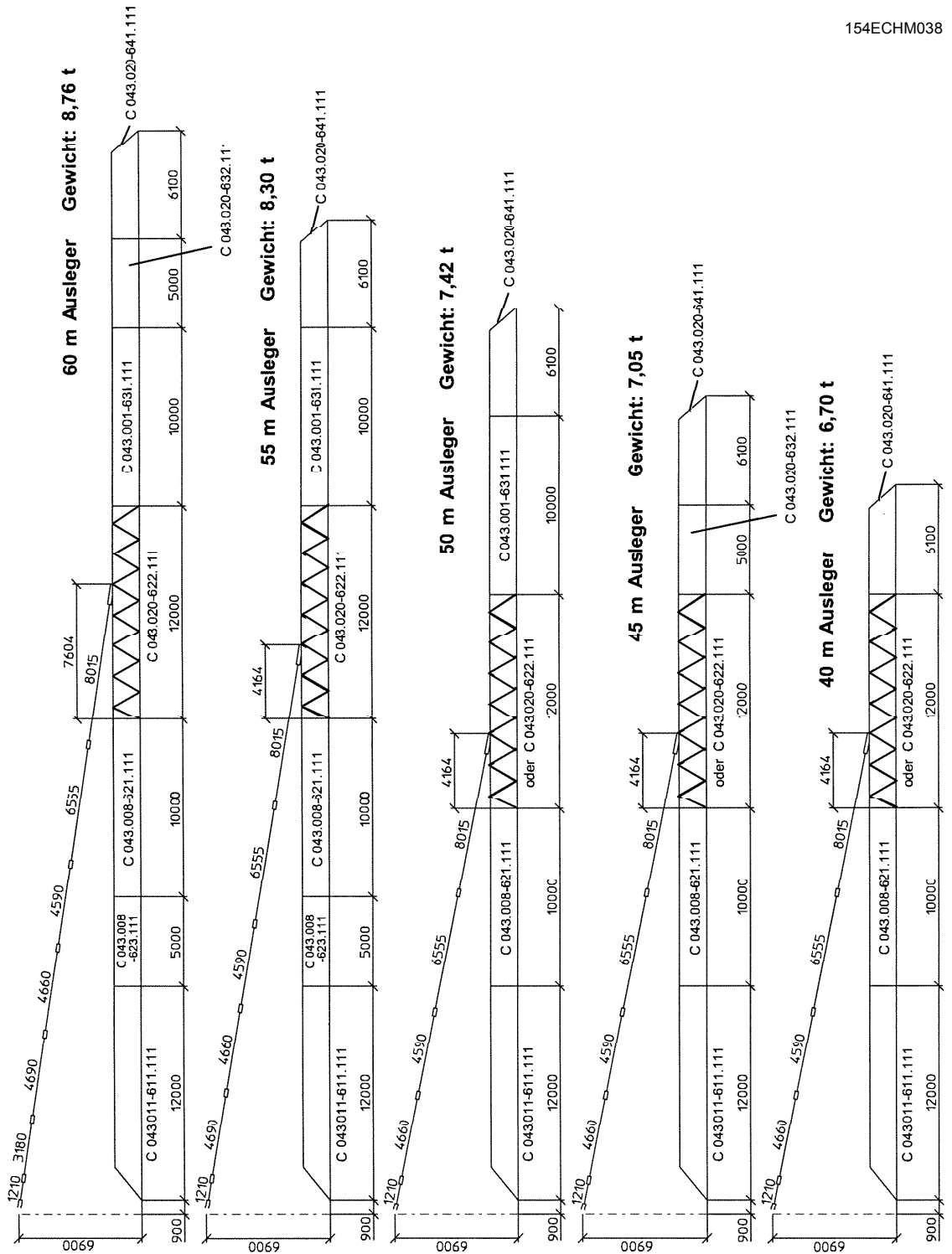
Fig. 6-15 Ausleger-Zusammenstellung und Ausleger-Abspannstangen
