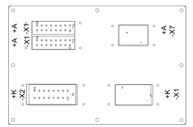
Ansicht SCHRANKAUSSENSEITE!
