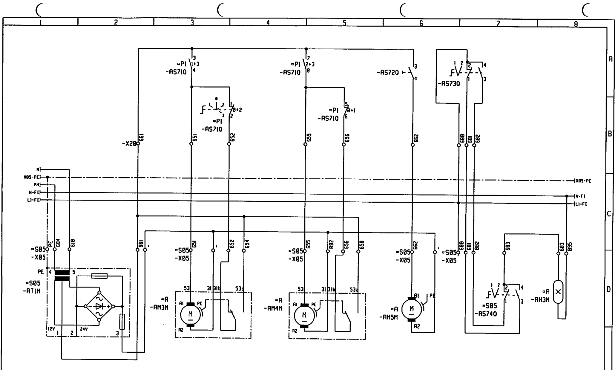
GLEICHRICHTERTRANSFORMATOR TRANSFORMER DC TRANSFORMATEUR DE REDRESSEUR
