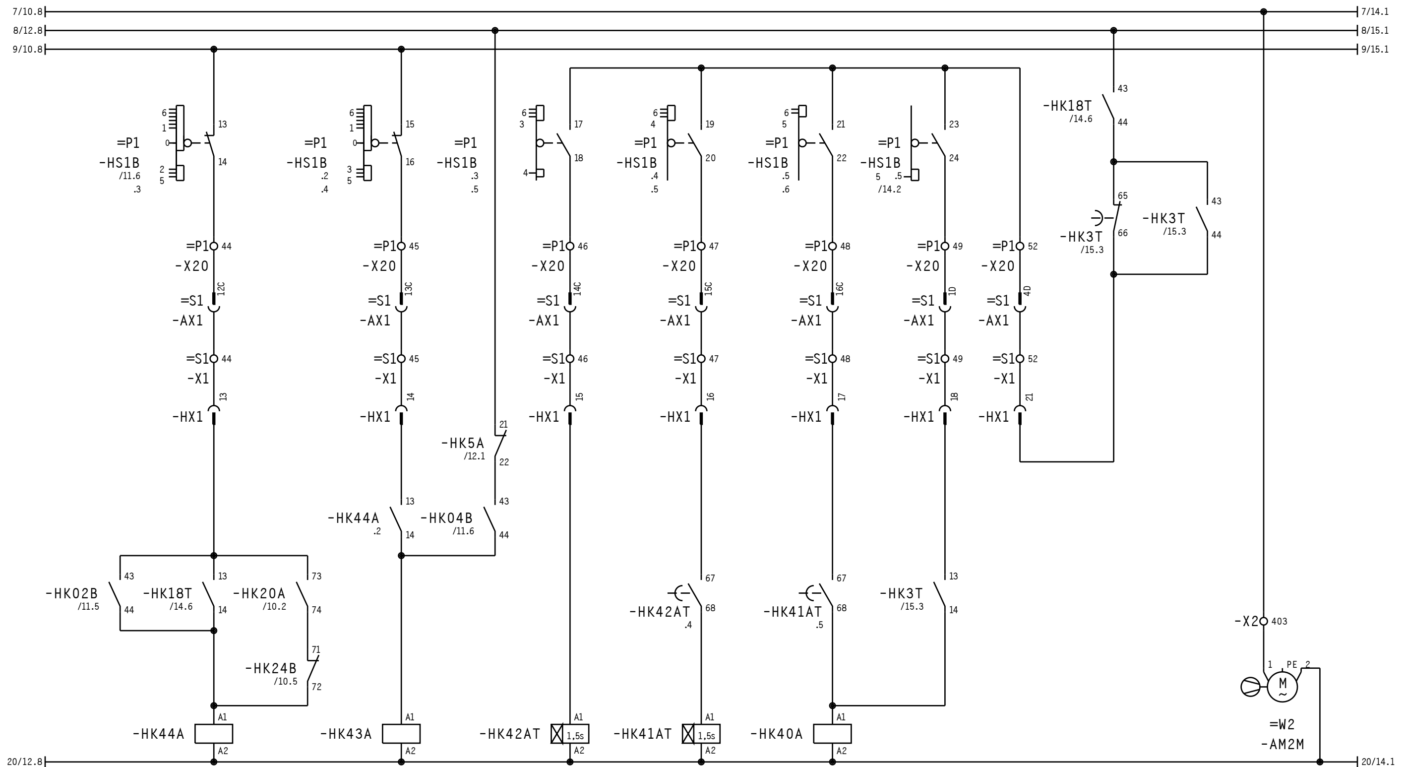
48-VENTILATOR 32-WIDERSTANDSSCHRANK
