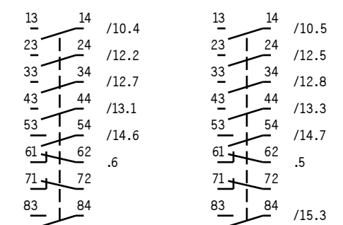
55-HEBEN 56-SENKEN
