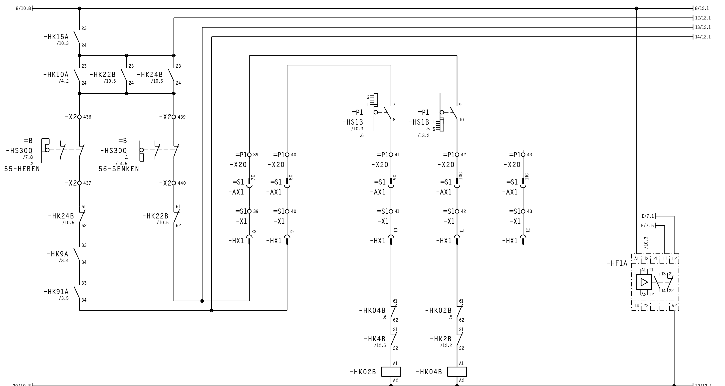
55-HEBEN 56-SENKEN
