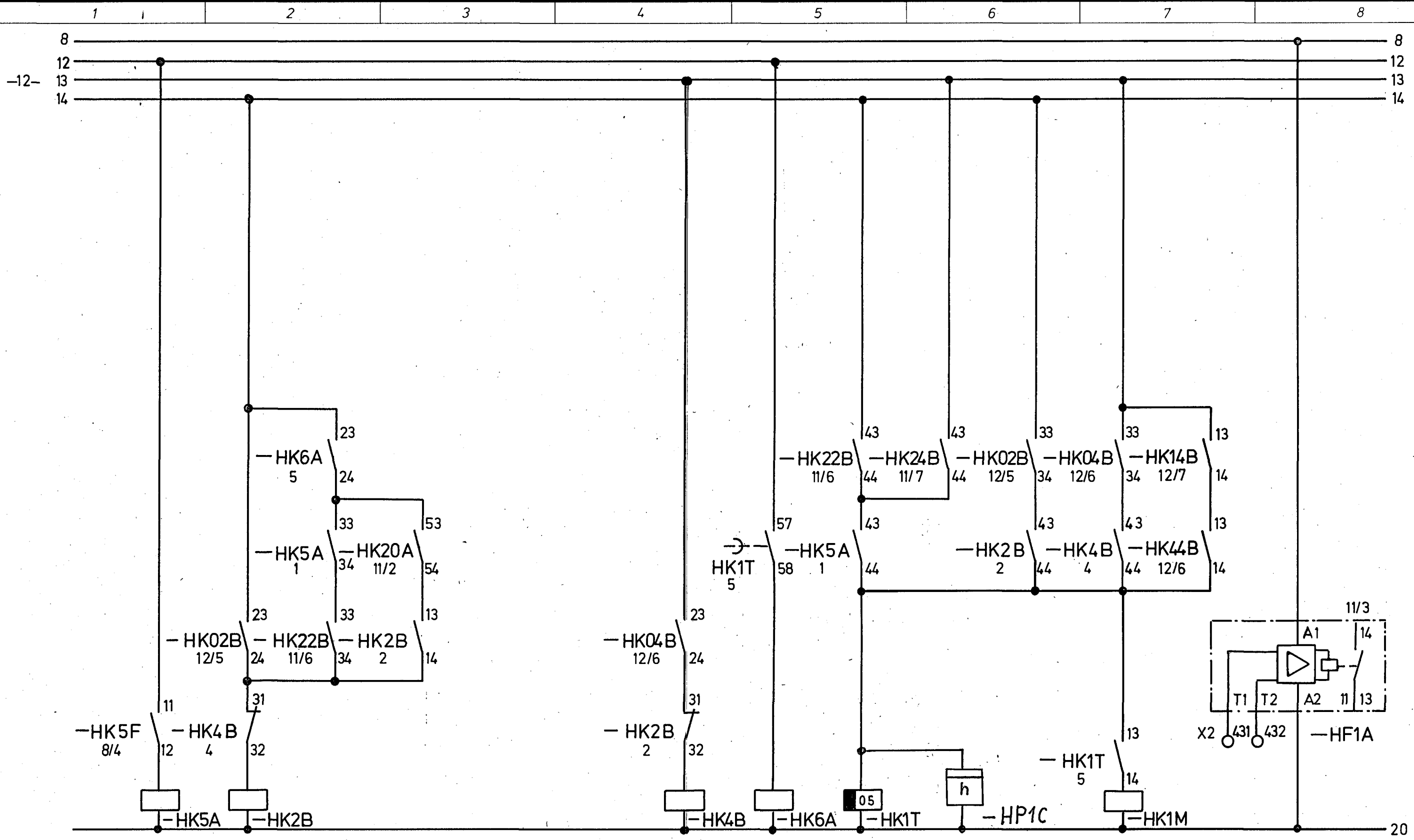
55-HEBEN
