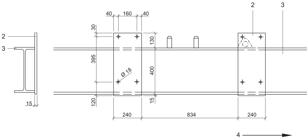
Lochbild der Werbetafelanbringung
