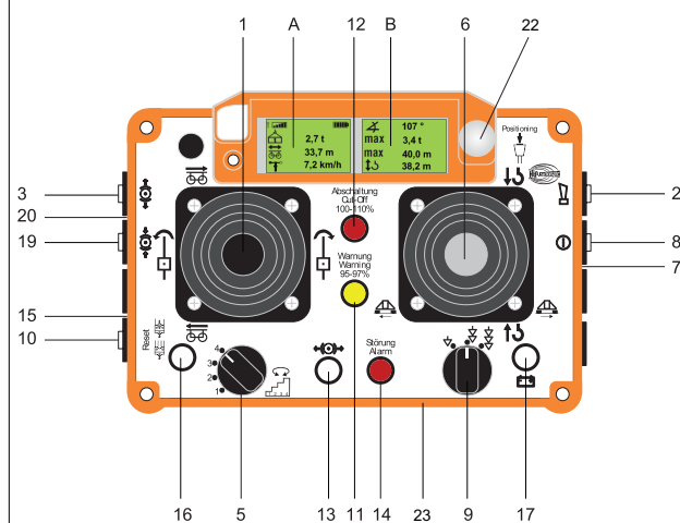
Funkfernsteuerung HBC radiomatic spectrum A
