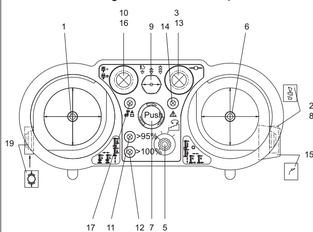
Funkfernsteuerung HETRONIC Nova
