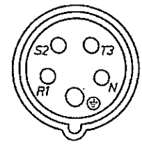
Ansicht von der Vorderseite der Kragensteckdose auf die Kontaktbuchsen
