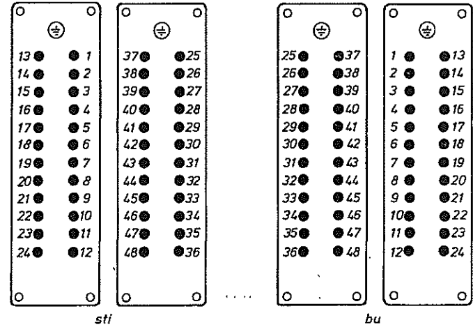
Ansicht - Anschlußseite
